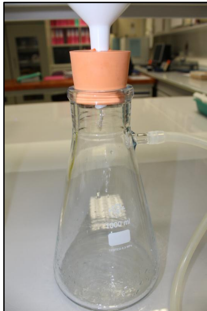
Figure 7 : la solution de lavage, plus l'eau osmosée ayant servi à rincer l'Erlenmeyer et à rincer les grains sont recueillies après filtration à 60 µm au fond de la première fiole à aspiration. Un volume de 300 à 400 mL peut être récupéré pour filtration dans le second dispositif équipé d'un filtre à 20 µm.
