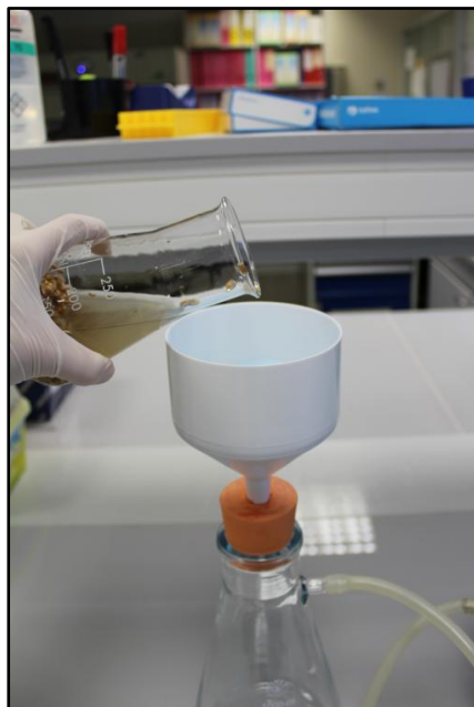
Figure 5 : la prise d'essai de 50 g et la solution de lavage sont versées sur le filtre de 60 µm, pendant que la fiole aspire.
