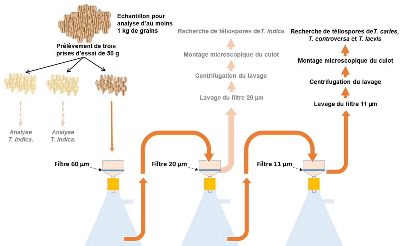
Schéma 2 : Principe général de la méthode de détection de T. caries , T. controversa et T. laevis , à la suite de la recherche de T. indica . Une seule des trois prises d'essai est analysée, par une étape supplémentaire de filtration à 11 µm.
