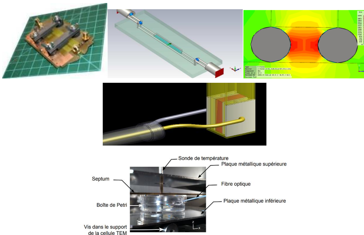
Figure 24 : Exemples d'applicateur de dimensions millimétriques entre 2 électrodes, pour des expositions in vitro .
