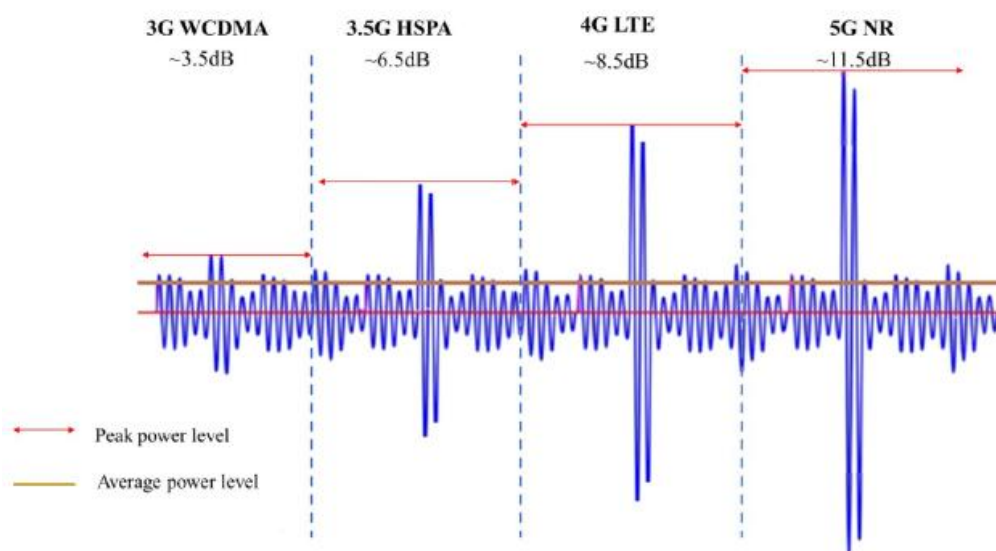
Figure 11 : Illustration du facteur de crête (ou Peak to Average Power Ratio – PAPR) suivant le type de modulation de signal radiofréquence
