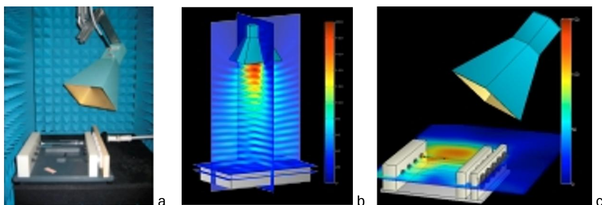
Figure 21 : (a) Exposition expérimentale avec un cornet et son pendant numérique avec calcul du champ dans un plan vertical (b) et horizontal (c).
