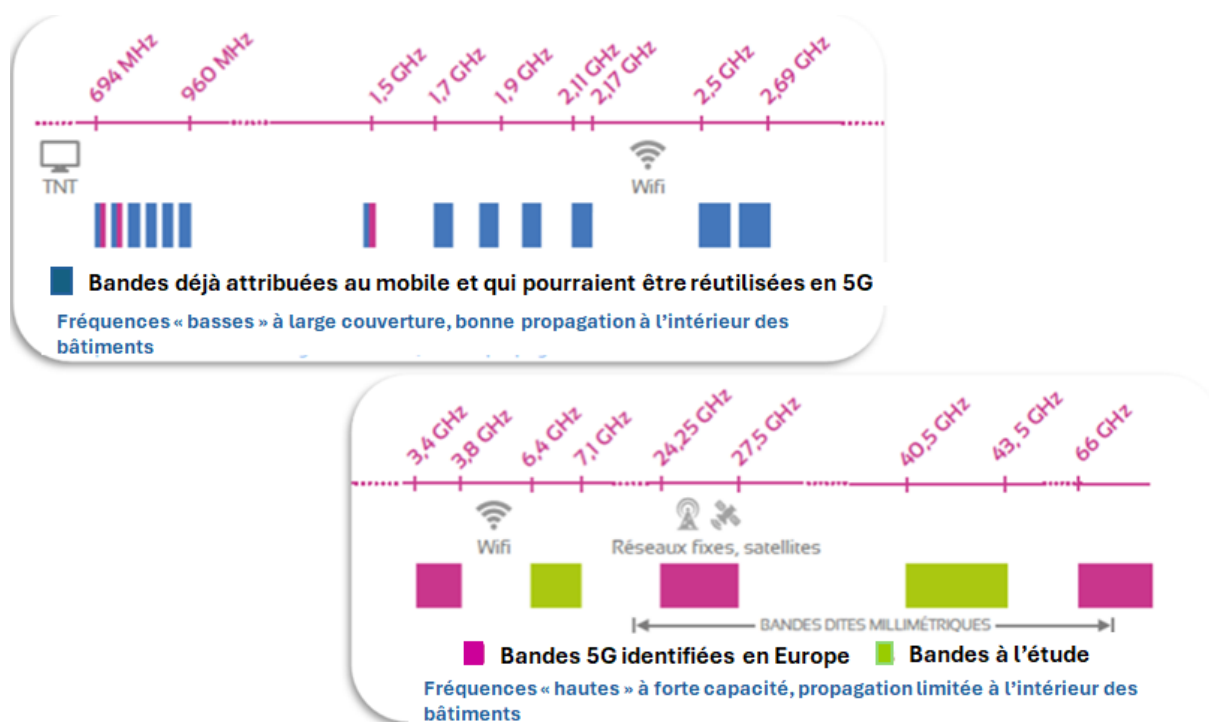
Figure 7 : Les bandes de fréquences (basses et hautes) attribuées au mobile et qui pourraient être utilisées en 5G.
