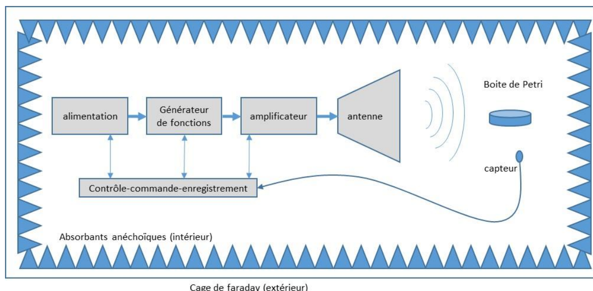
Figure 17 : Représentation du principe d'une chaîne d'émission générique assurant une exposition reproductible en espace libre.
