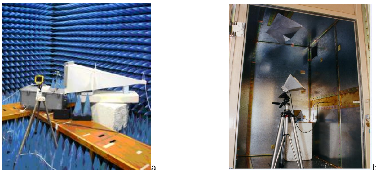
Figure 18 : Exemples de montages d'essais en chambre anéchoïque (a) et en chambre réverbérante à brassage de modes (b).
