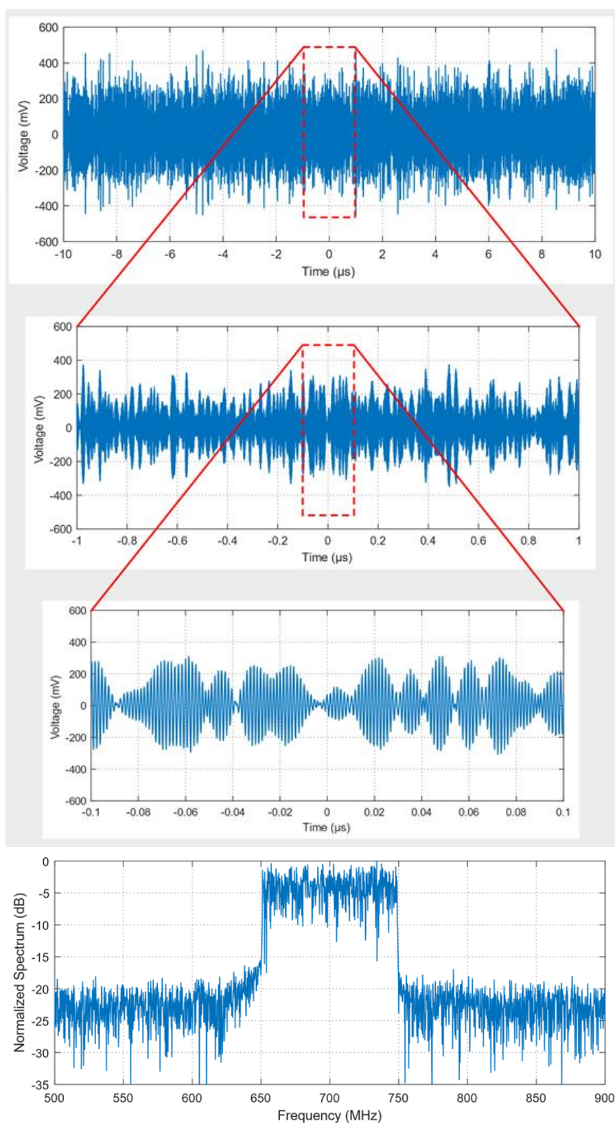
Figure 10 : L'évolution temporelle d'un signal 5G, à différentes échelles, ainsi que la bande passante sur le spectre associé 29 .
