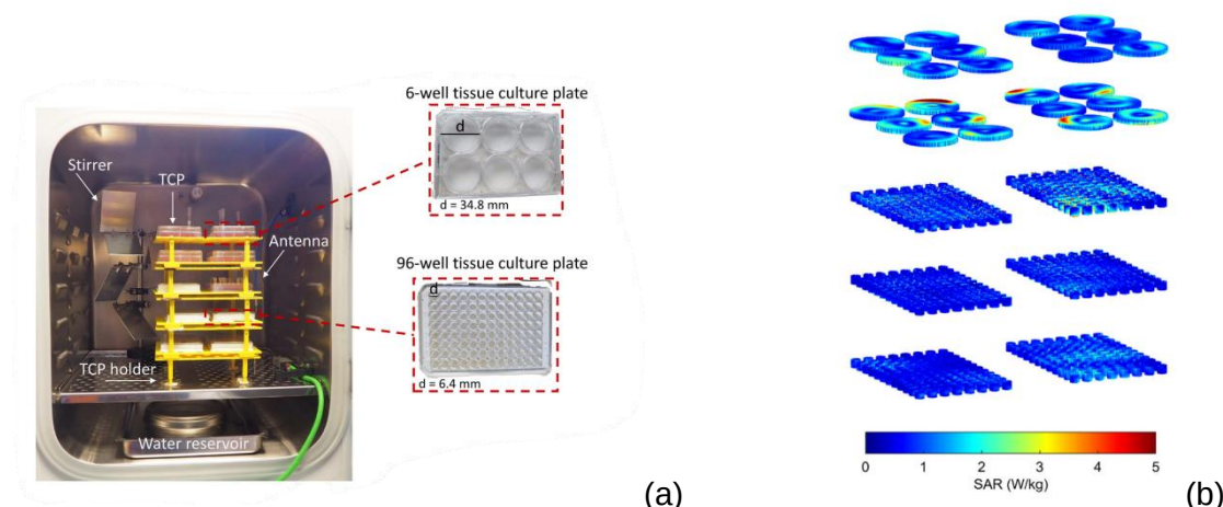
Figure 20 : (a) Exposition expérimentale in vitro de plaques 6 puits et de plaques 96 puits dans une chambre réverbérante à brassage de mode et (b) : son pendant numérique avec calcul de DAS.
