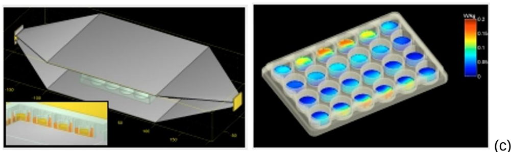
Figure 22 : Exemples d'une cellule TEM pour des essais in vivo ou in vitro (a) et ses pendants numériques in vivo (b) et in vitro (c)
