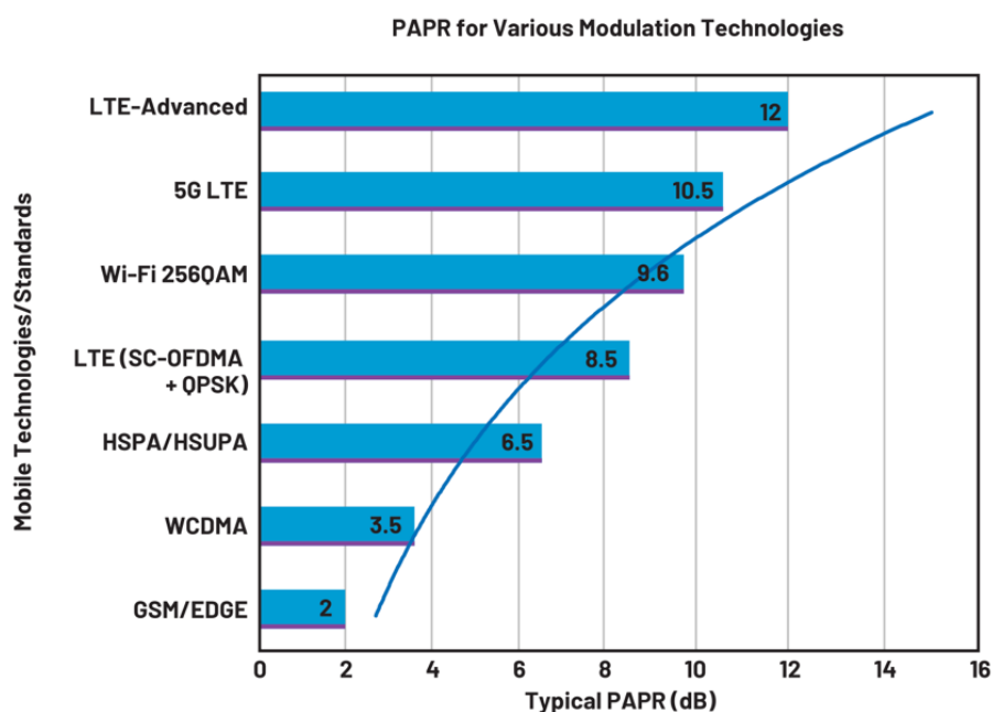
Figure 12 : Niveau du facteur crête suivant le type de modulation de signal radiofréquence.
