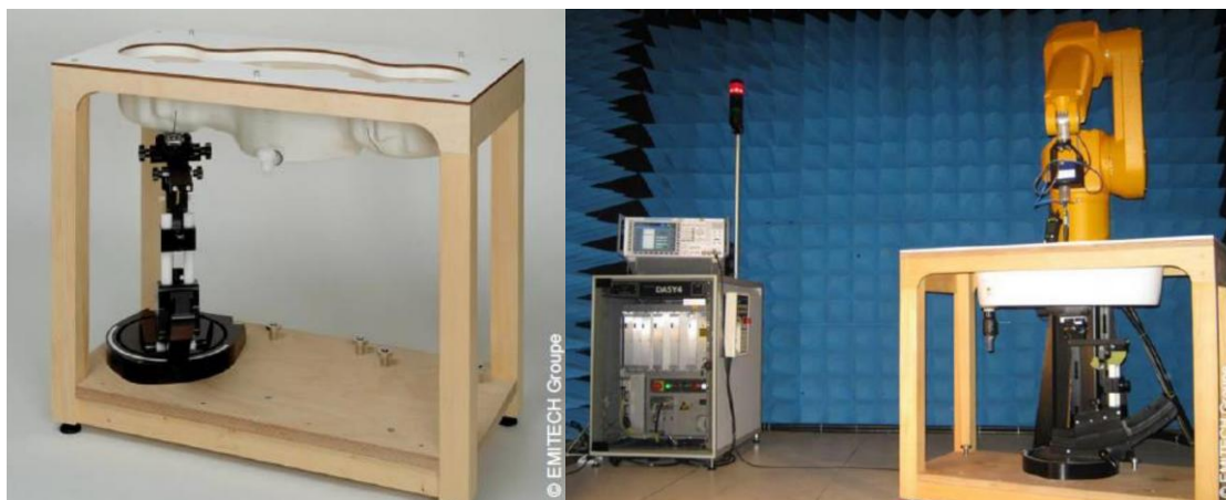
Figure 28 : Illustration de mesures dans une tête à proximité d'un téléphone mobile.
