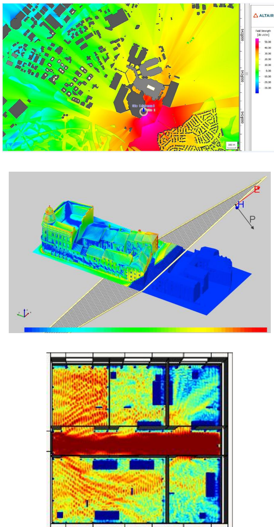
Figure 16 : Illustrations qualitatives des possibilités de simulation numérique à l'échelle d'une ville (en haut), d'un quartier de ville (au centre) et dans un bâtiment (en bas).
