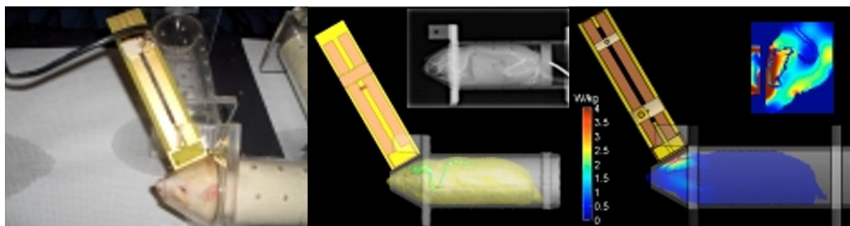
Figure 25 : Exemple d'un applicateur pour des expositions in vivo sur la tête d'un rongeur.
