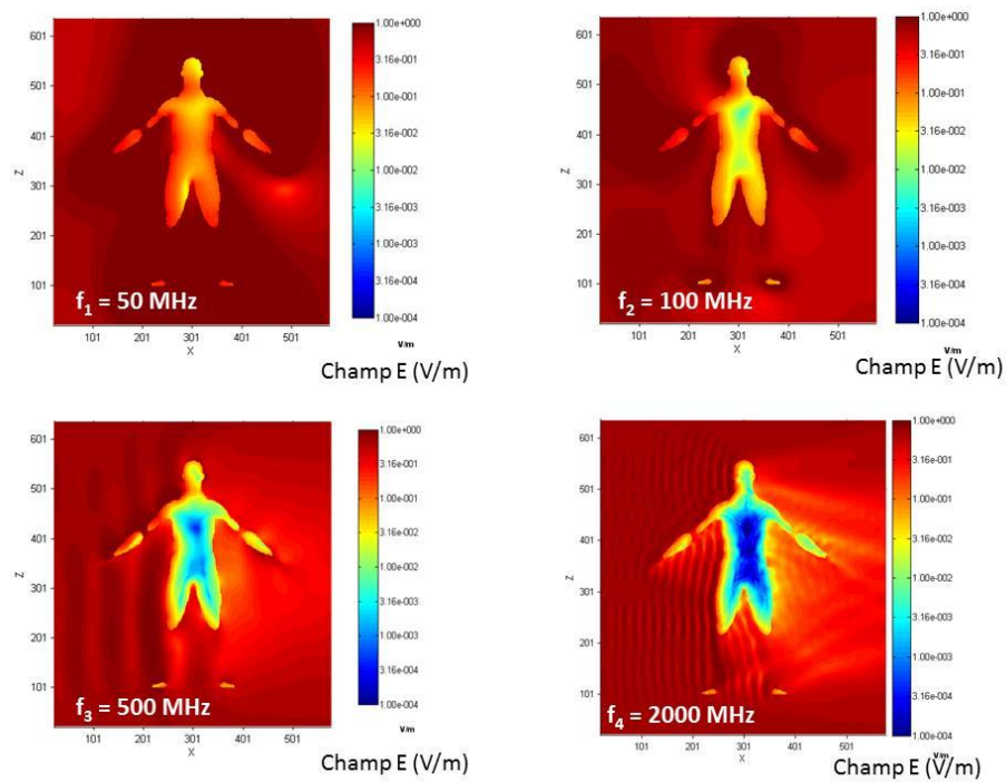
Figure 26 : Illustration du champ électrique dans le corps d'un modèle homogène.
