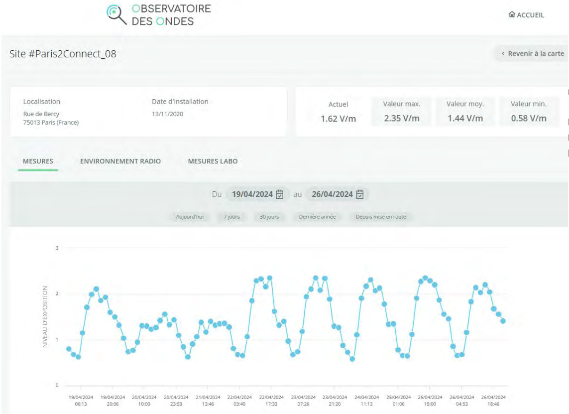
Figure 12 : Illustration de la surveillance de l'environnement électromagnétique, variation du champ électrique (V/m) sur une semaine (source Observatoire des ondes, Paris).
