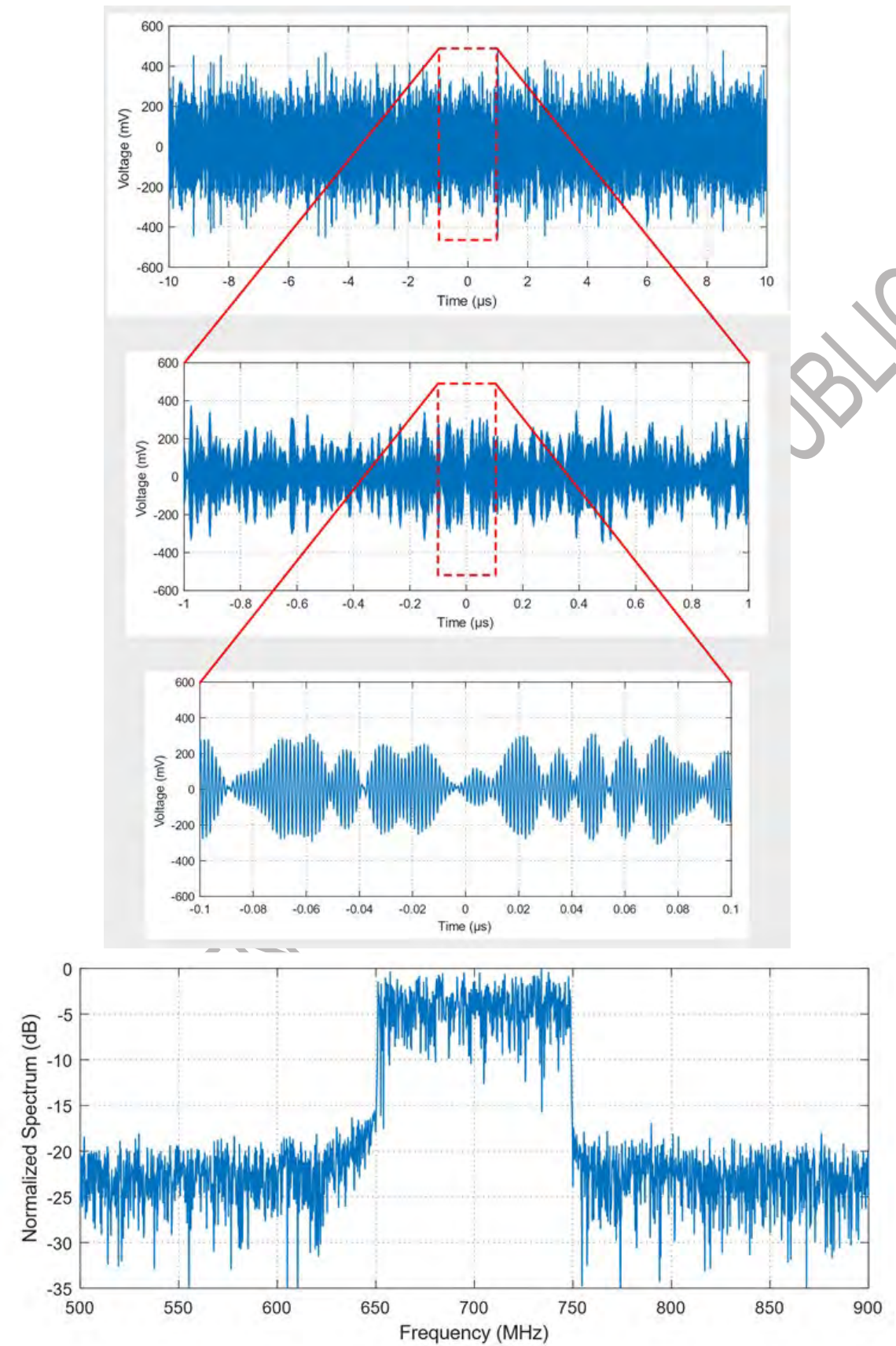
Figure 10 : L'évolution temporelle d'un signal 5G, à différentes échelles, ainsi que la bande passante sur le spectre associé.
