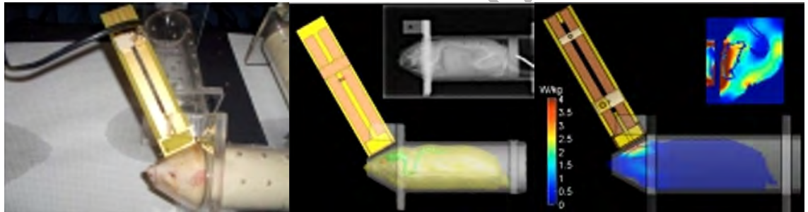
Figure 23 : Exemple d'un applicateur pour des expositions in vivo sur la tête d'un rongeur. Source : XLIM.
