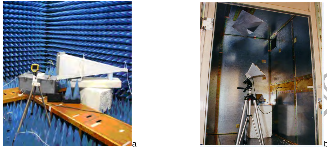
Figure 16 : Exemples de montages d'essais en chambre anéchoïque (a) et en chambre réverbérante à brassage de modes (b).
