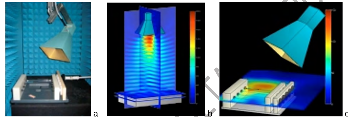
Figure 19 : (a) Exposition expérimentale avec un cornet et son pendant numérique avec calcul du champ dans un plan vertical (b) et horizontal (c) (source : XLIM).
