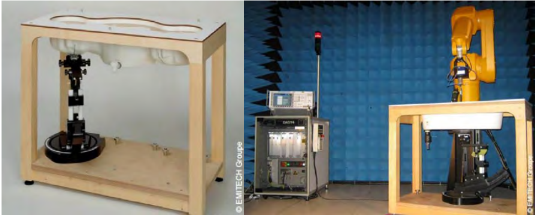
Figure 26 : Illustration de mesures dans une tête à proximité d'un téléphone mobile. Source : EMITECH.
