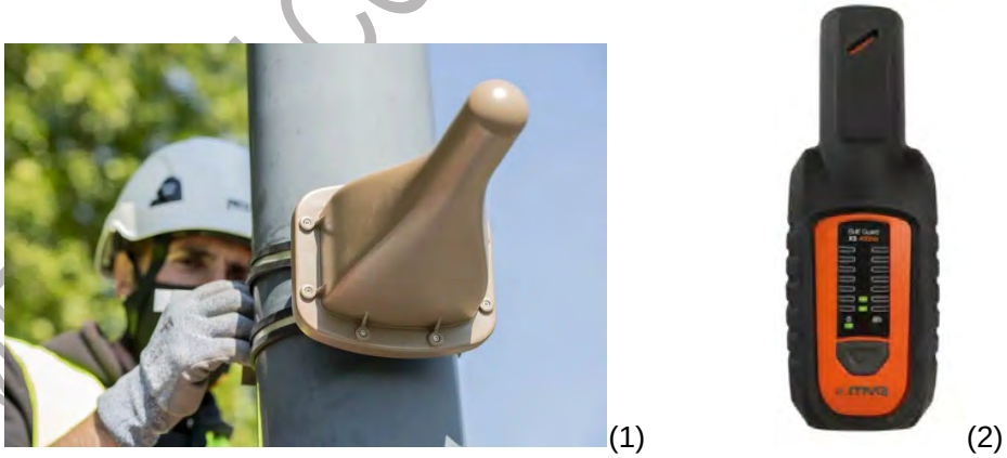
Figure 13 : Illustration d'outils de mesure de champ électromagnétique (1) : capteur fixe WAVE-001 de EXEM, et d'un exposimètre portable (2) : EME Guard XS 1 MHz – 40 000 MHz de MVG.
