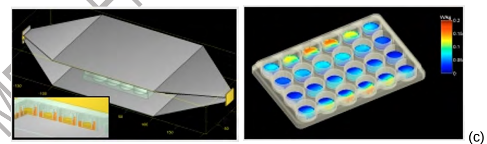
Figure 20 : Exemples d'une cellule TEM pour des essais in vivo ou in vitro (a) et ses pendants numériques in vivo (b) et in vitro (c)
