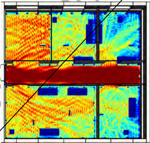
Figure 14 : Illustrations qualitatives des possibilités de simulation numérique à l'échelle d'une ville (en haut), d'un quartier de ville (au centre) et dans un bâtiment (en bas).
