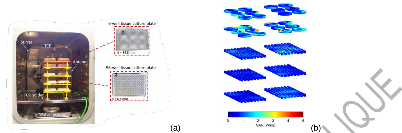
Figure 18 : (a) Exposition expérimentale in vitro de plaques 6 puits et de plaques 96 puits dans une chambre réverbérante à brassage de mode et (b) : son pendant numérique avec calcul de DAS (source : XLIM).
