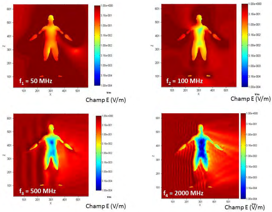
Figure 24 : Illustration du champ électrique dans le corps d'un modèle homogène.
