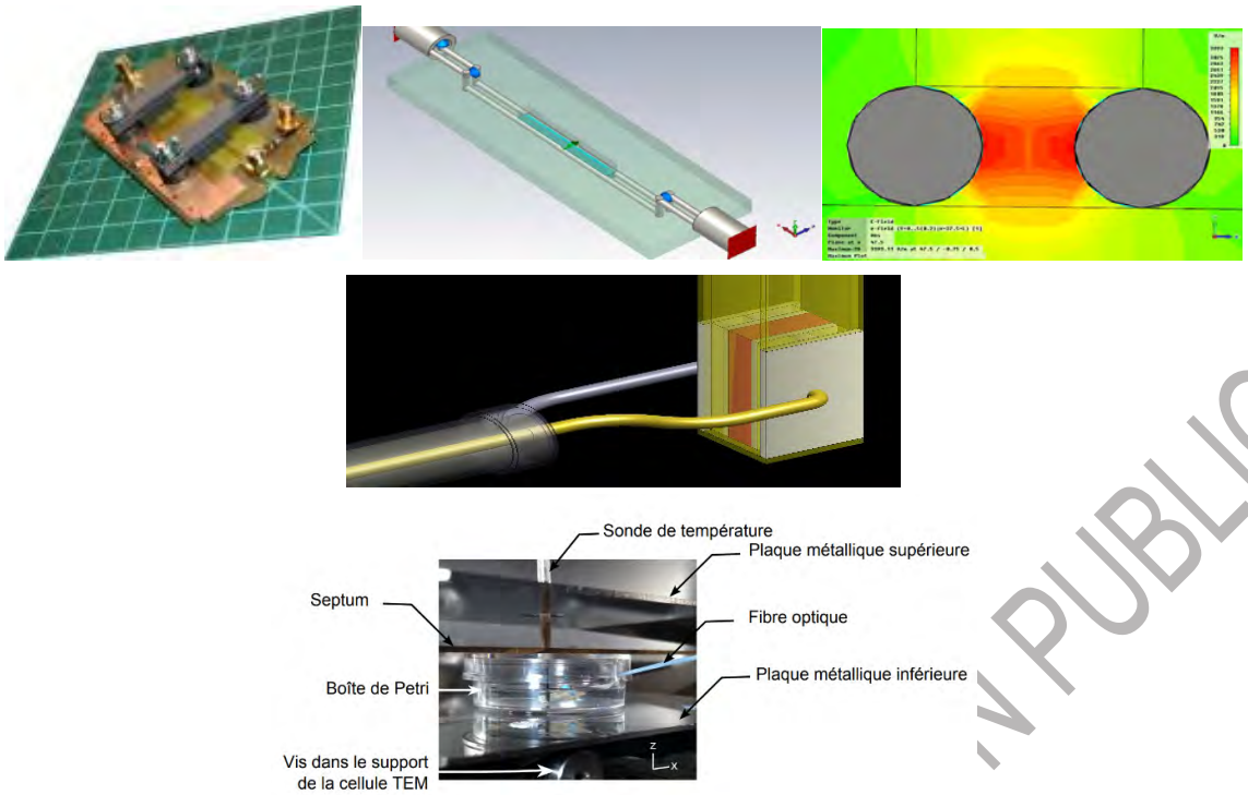
Figure 22 : Exemples d'applicateur de dimensions millimétriques entre 2 électrodes, pour des expositions in vitro . Sources : CEA et XLIM.
