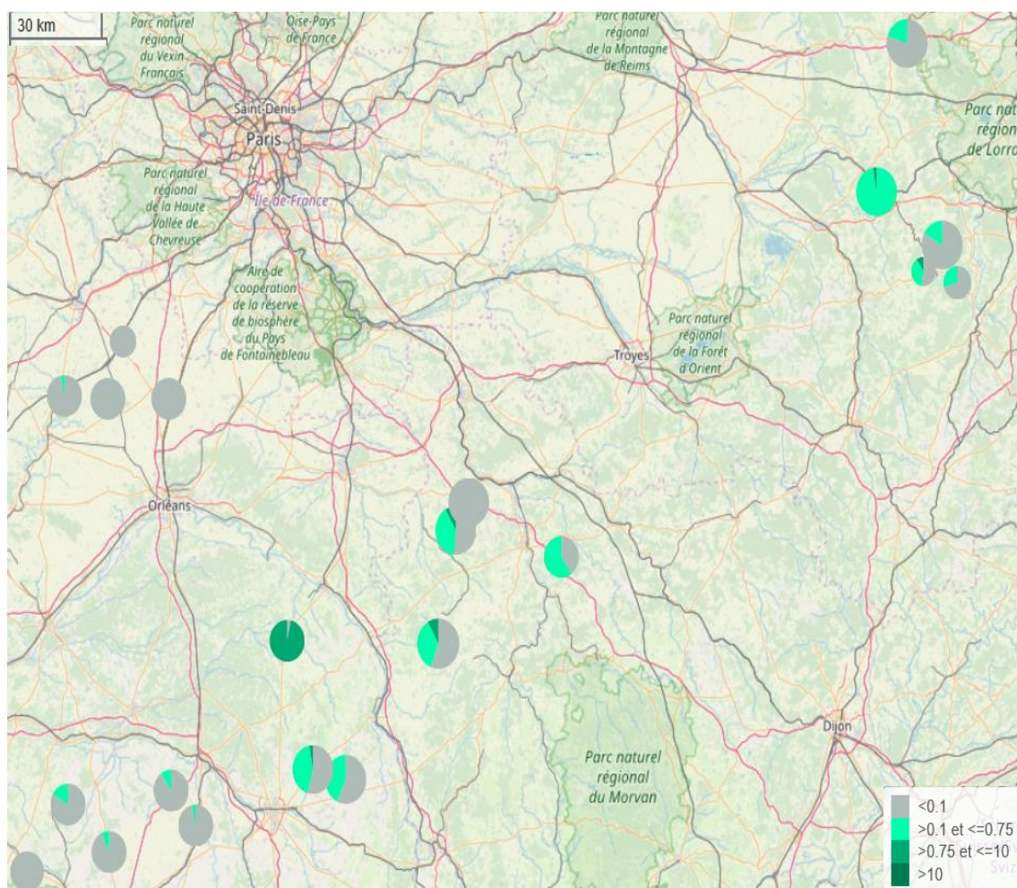
Figure 2 : Répartition des concentrations (µg/L) en métabolite BH 479-8 (métazachlore ESA) mesurées dans chaque puits sur la période 2010-2017 (la taille du camembert est fonction du nombre d'analyses disponibles)
